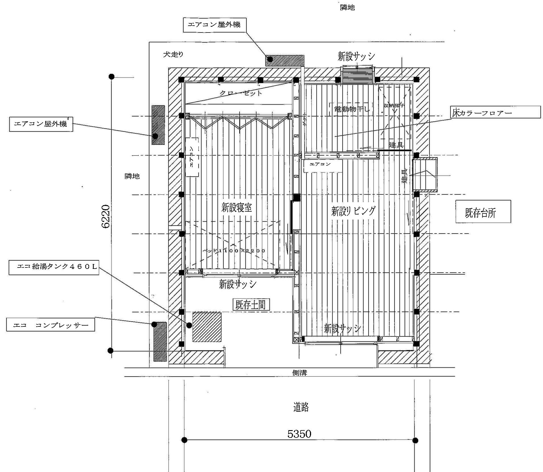
土蔵改装平面図
